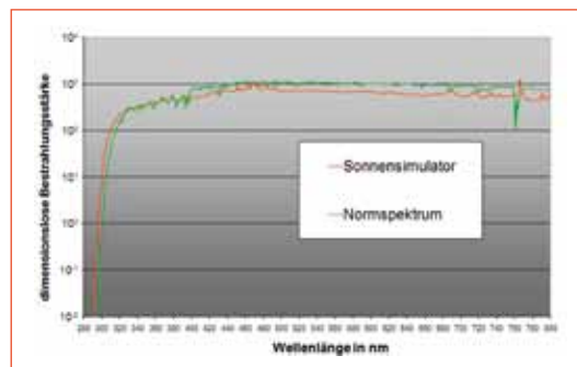
Abb. 8: Spektrum des Sonnensimulators im Vergleich zum ASTM-Normspektrum
