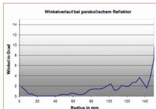
Abb. 3: Winkelverteilung der Strahlen im primären Filter bei 30 cm Abstand zum Reflektor
